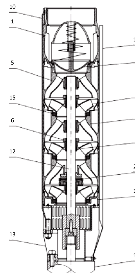
Вид в разрезе SJ95 (насосная часть)
